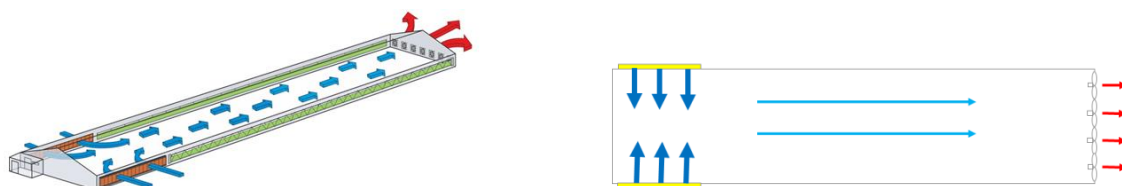
Beispiel einer Tunnellüftung, die sich insbesondere bei hohen Temperaturen bewährt hat (Abbildung links: seitliche Ansicht und Abbildung rechts: in der Aufsicht).
